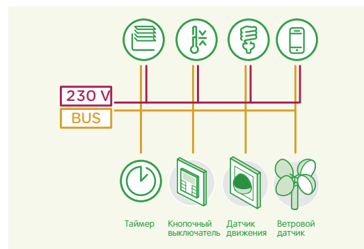
Интеллектуальное решение KNX: шина выполняет все функции управления, максимальная гибкость
